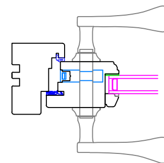
Door Typ. Jamb (opening)
