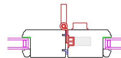
Door Leafs
