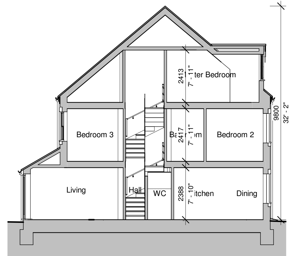
Section A-A 1 : 100
