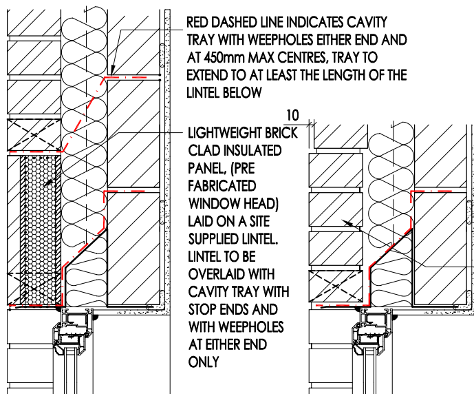
4 COURSE VOUSIOR DETAIL
