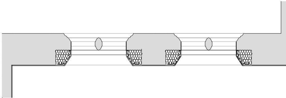
Plan Section 02 - 1:50
