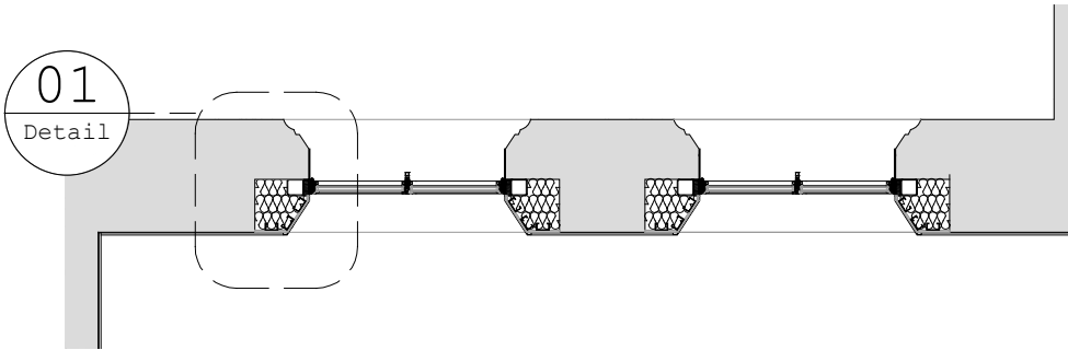
Plan Section 01 - 1:50
